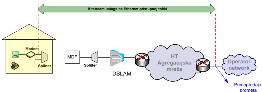
Slika 3. Veleprodajni širokopoljاسni pristup za pružanje Internet usluge na Ethernet razini u slučaju kada Krajnji korisnik ostvaruje Osnovni pristup mreži putem usluge HT-a.
