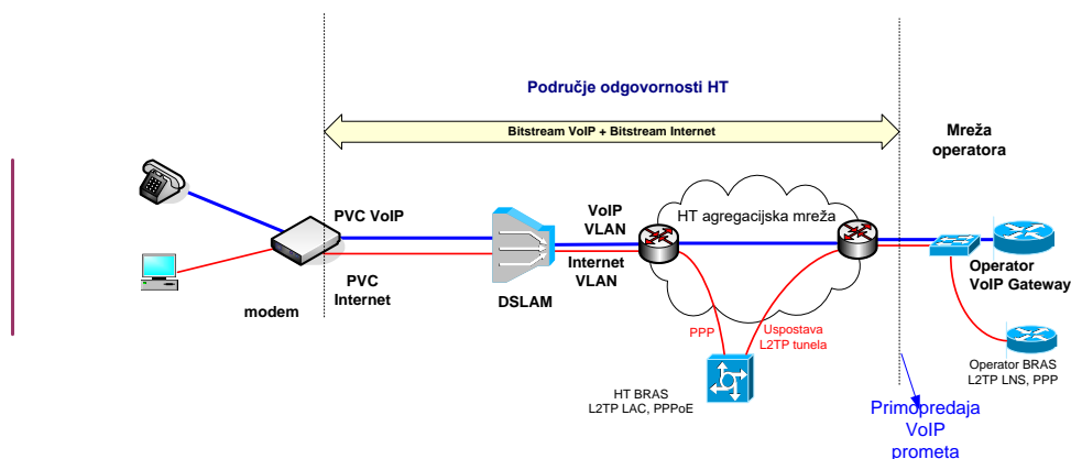
Slika 12. Realizacija posebnog virtualnog kanala za VoIP uslugu preko ADSL/VDSL pristupa (kod VDSL pristupa između modema i DSLAM-a koristi se dogovarajući VLAN)
