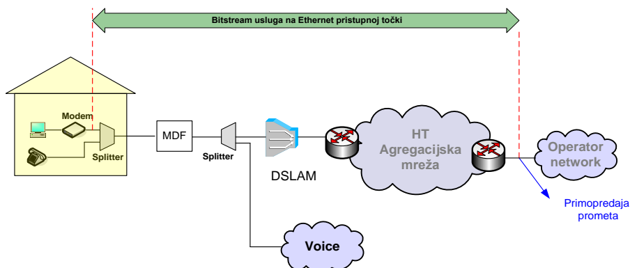
Slika 3. Veleprodajni širokopoljاسni pristup za pružanje Internet usluge na Ethernet razini u slučaju kada Krajnji korisnik ostvaruje Osnovni pristup mreži putem usluge HT-a.
