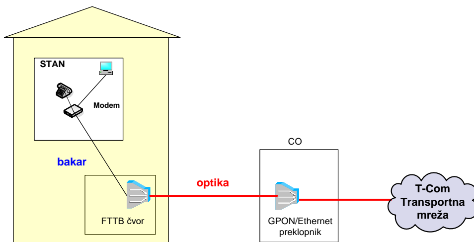
Slika 35. Način realizacije FTTB koncepta sa VDSL17a tehnologijom u pristupnoj mreži
